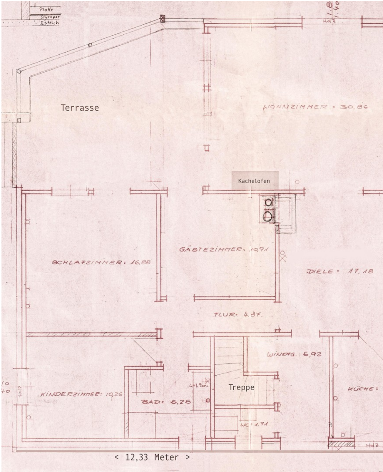
Grundriss Erdgeschoss
