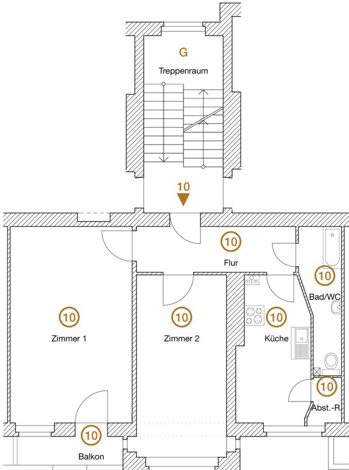
Grundriss 3. OG mitte
