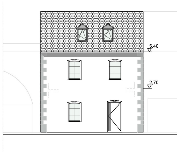
Ansicht Innenhof
