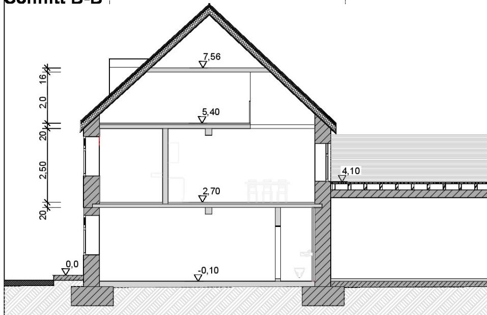
Schnitt B-B
