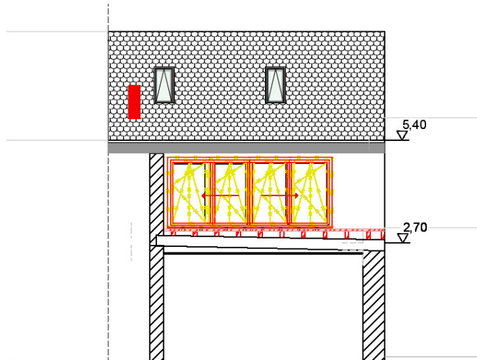
Ansicht Innenhof
