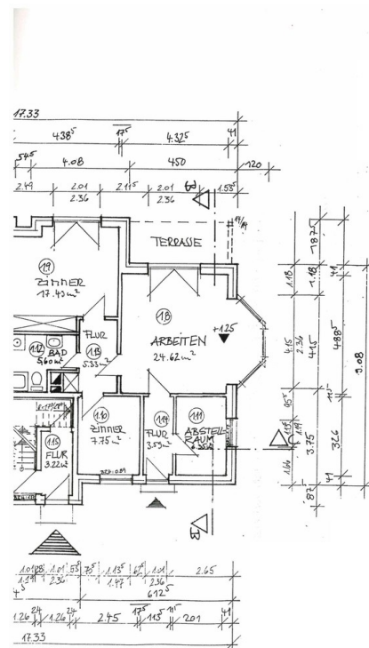
Grundriss
