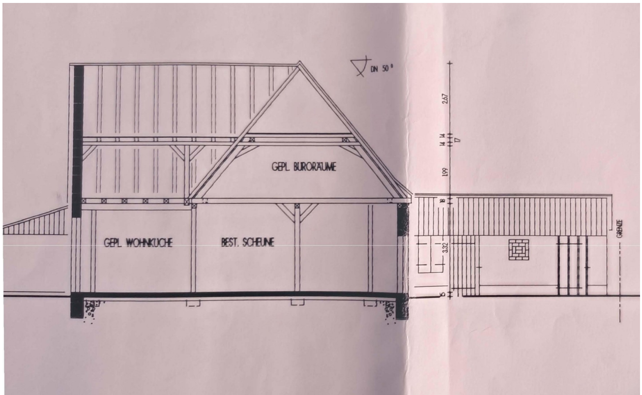
Längsschnitt
