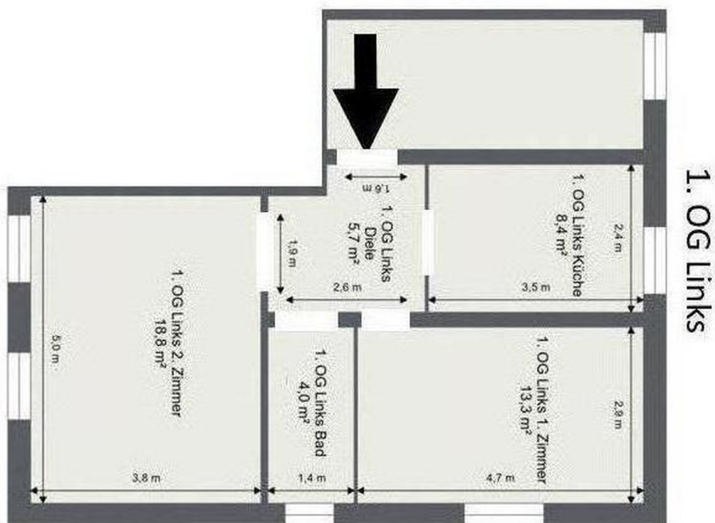
Grundriss nach Bauzeichnung
