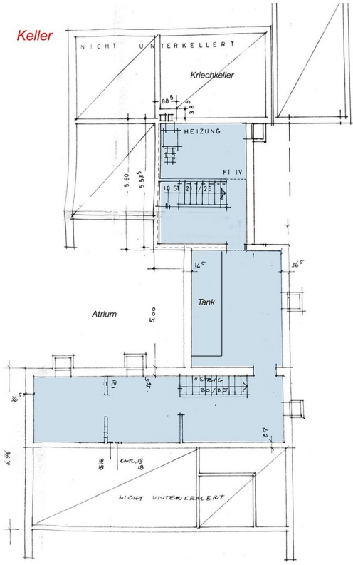
Keller
