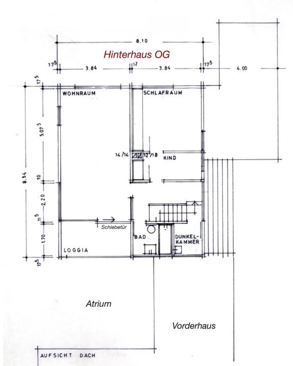
Hinterhaus OG
