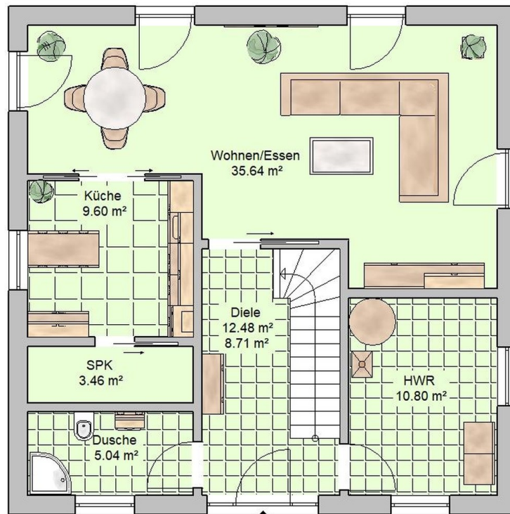
Grundriss Stadtvilla EG
