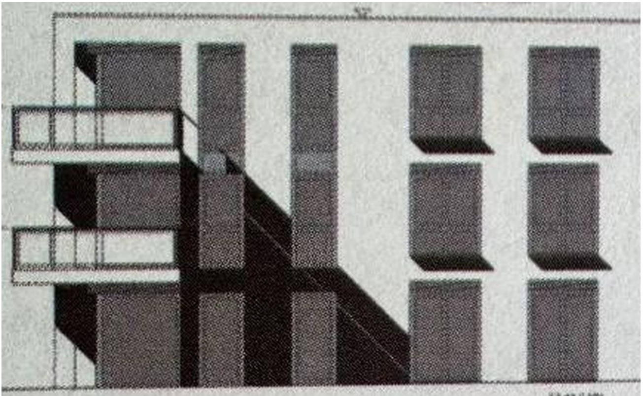
Ansicht 4
