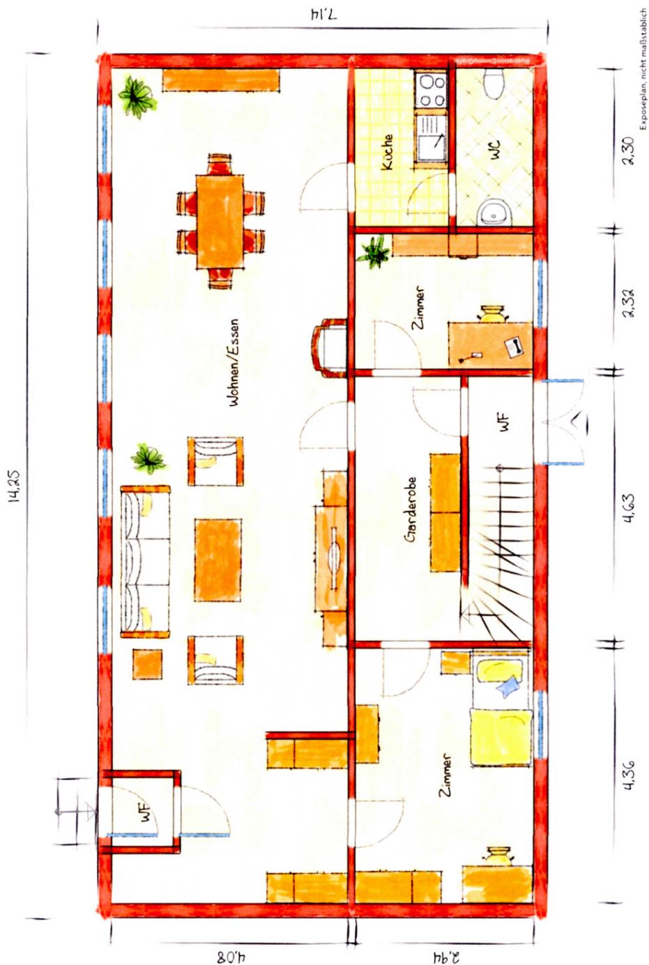
Erdgeschoss
