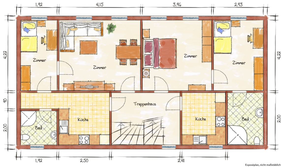
Obergeschoss
