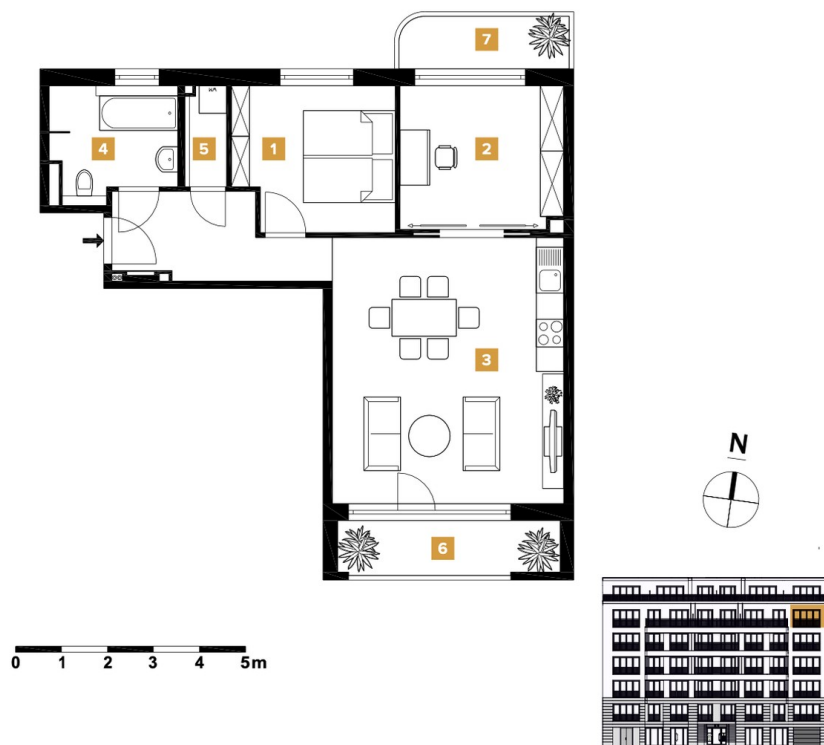
Grundriss H9-09
