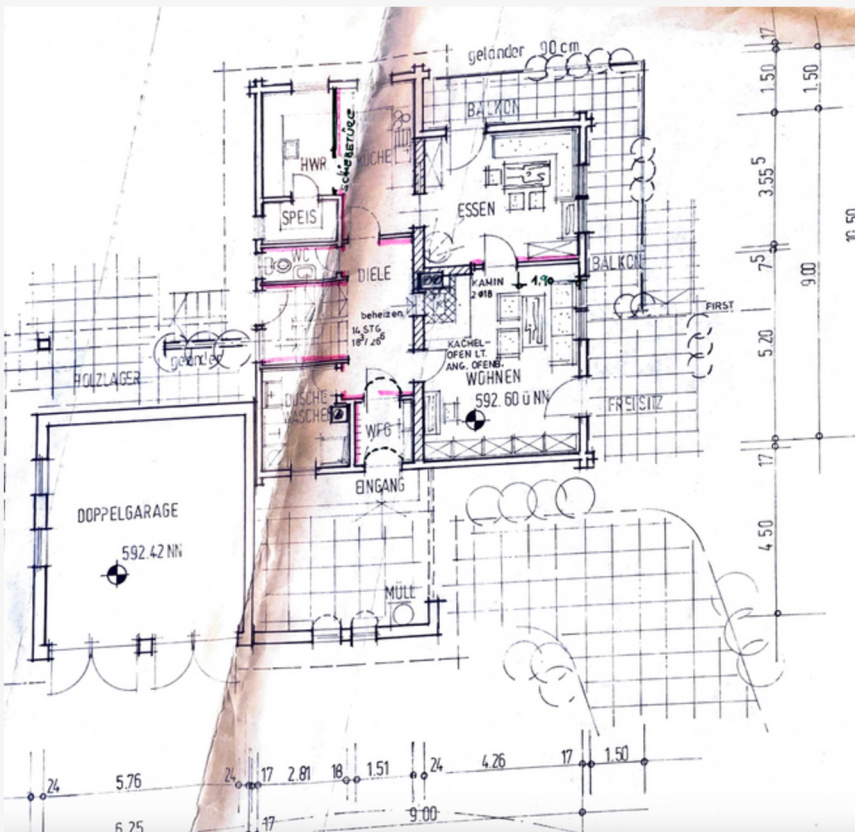
ERDGESCHOSS
