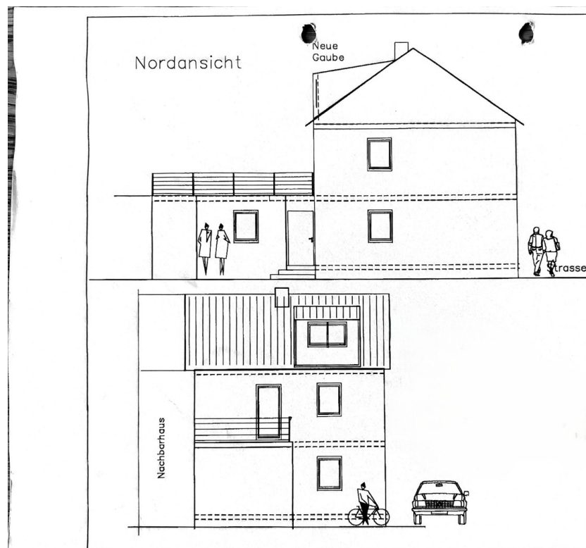
Vorderansicht Plan
