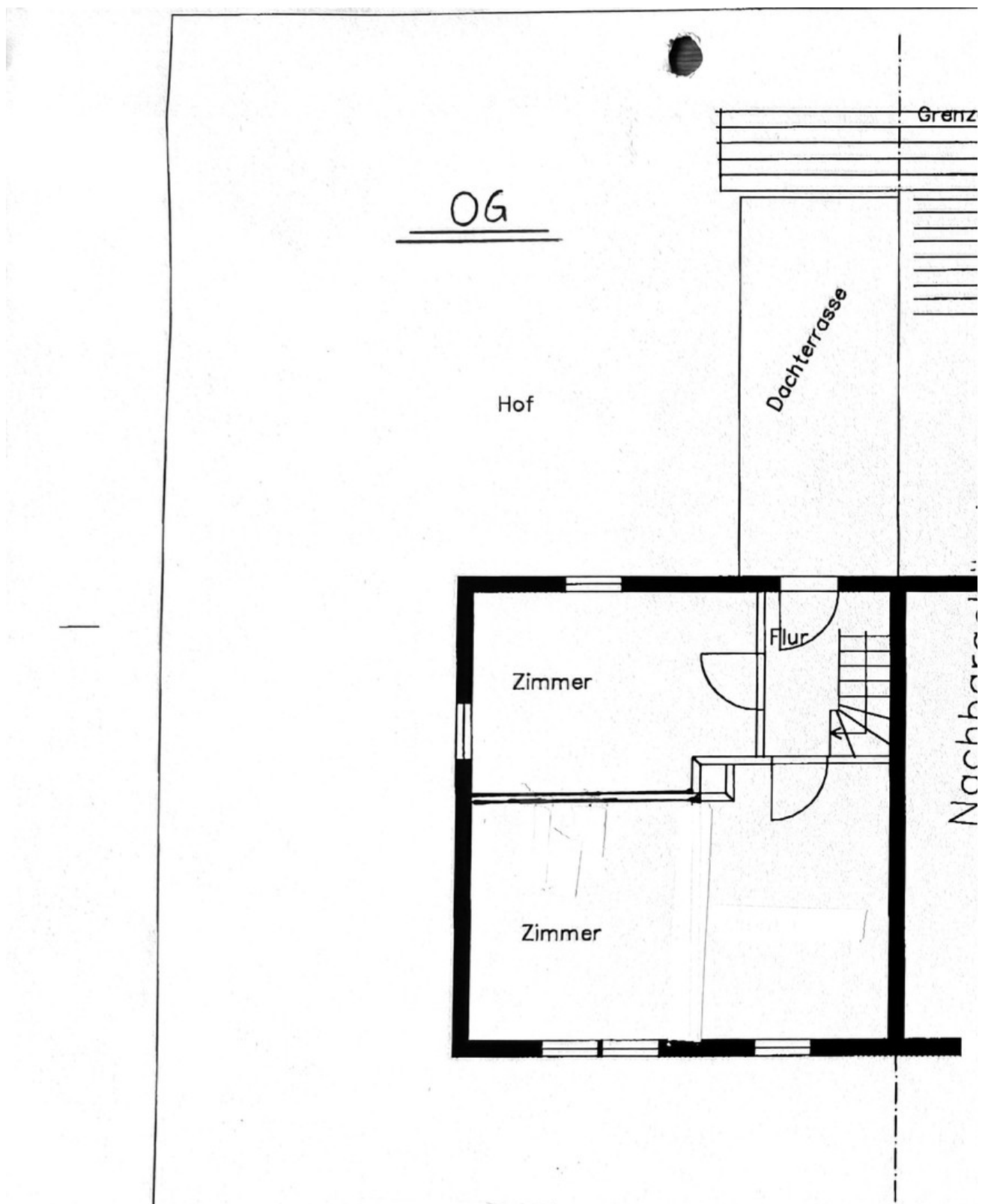
Grundriss OG
