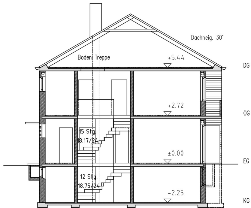
Schnitt Haus
