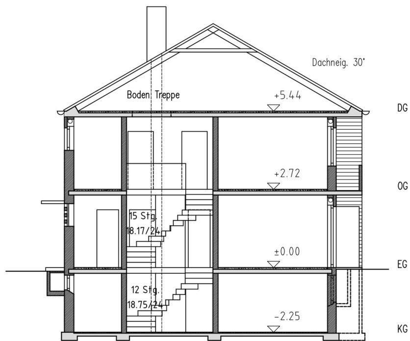
Schnitt Haus
