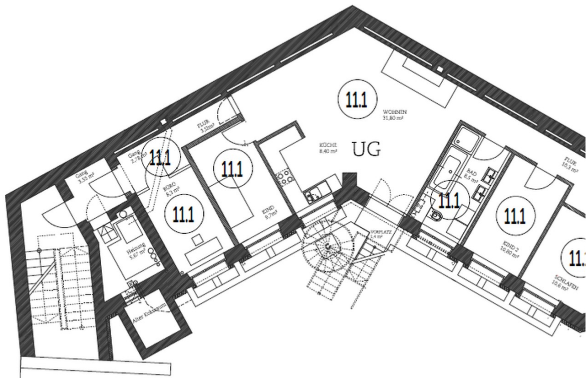
Grundriss
