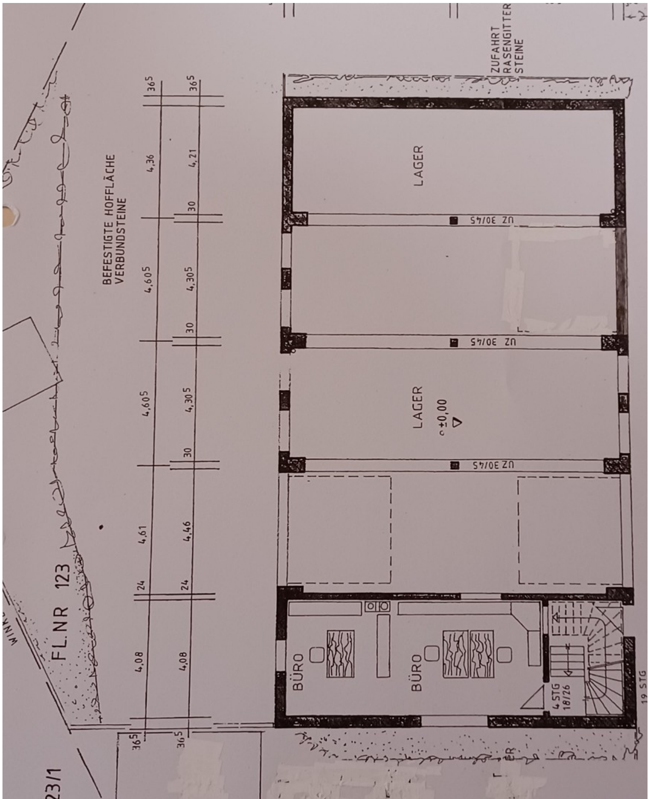
Grundriss Halle u. Büro
