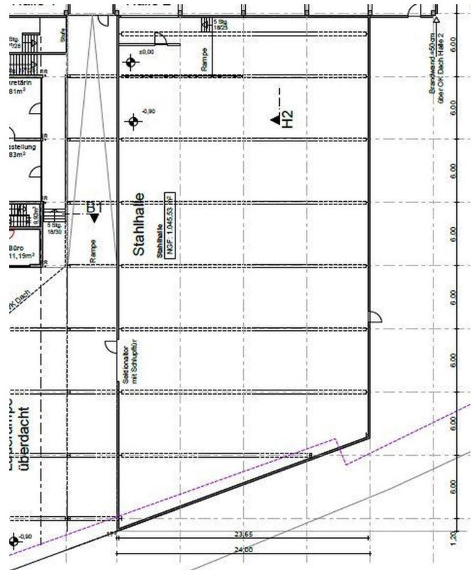
Grundriss Stahlhalle
