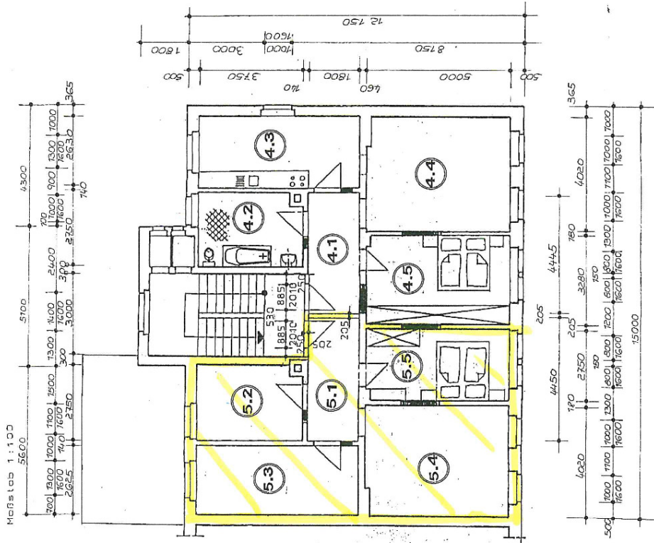
Grundriß 2. Obergeschoß
