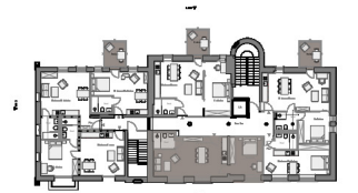
Übersichtsplan Ebene E3
