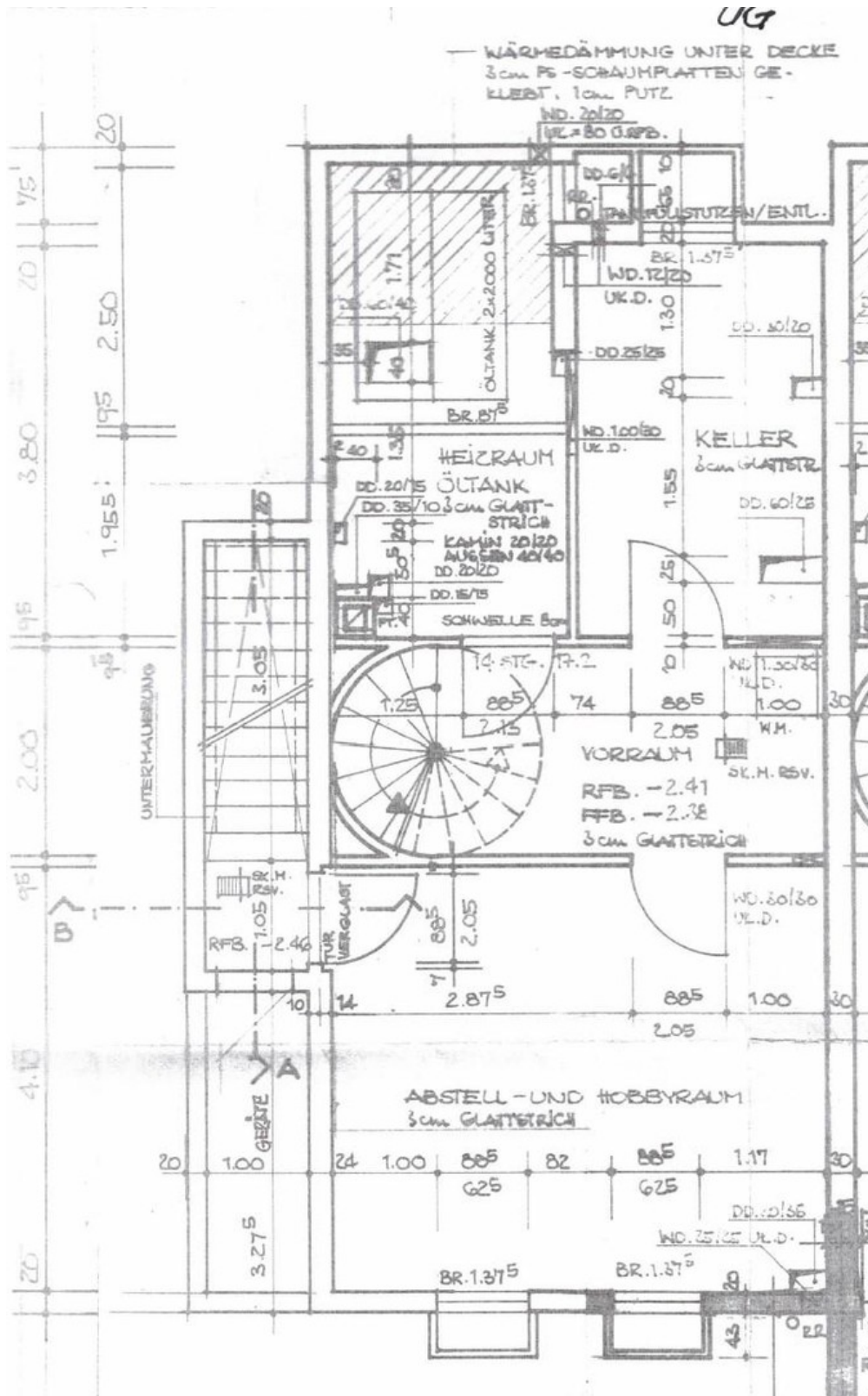
Untergeschoss
