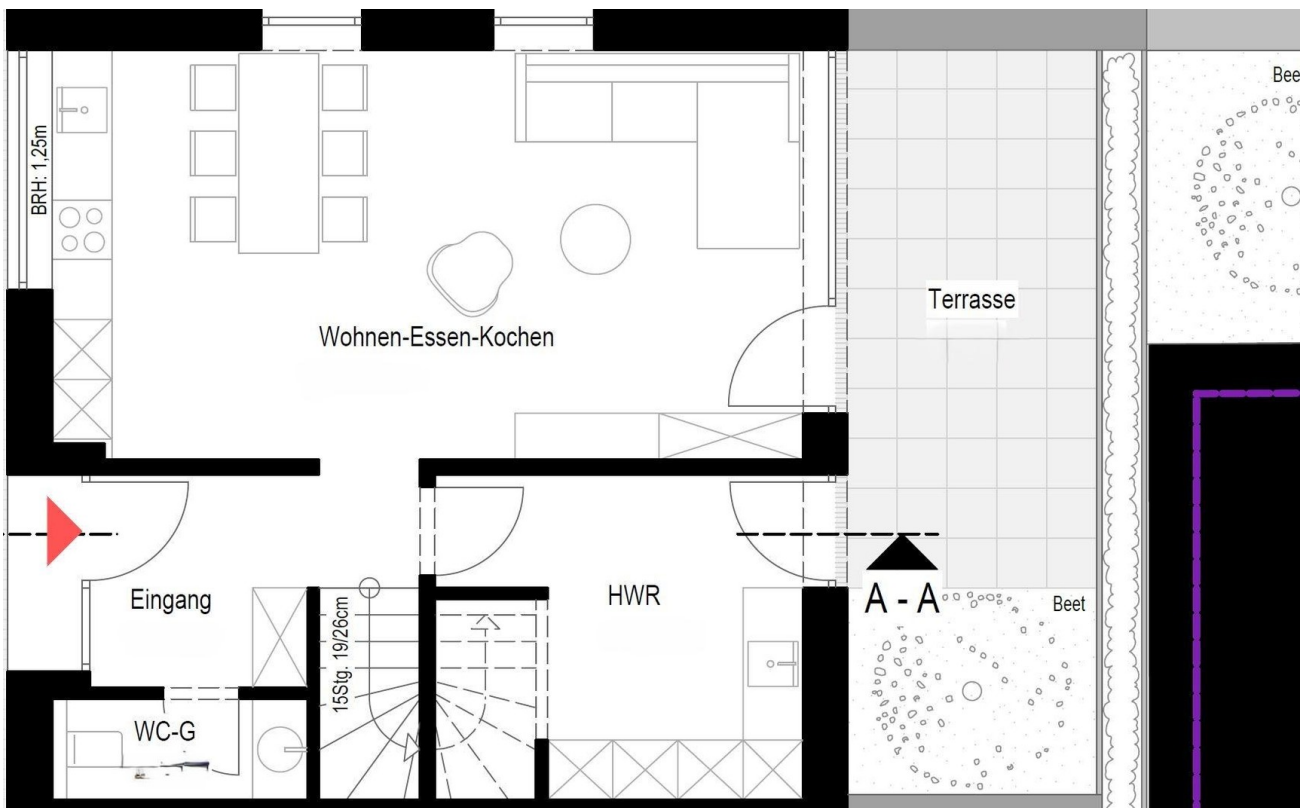
Grundriss Erdgeschoss
