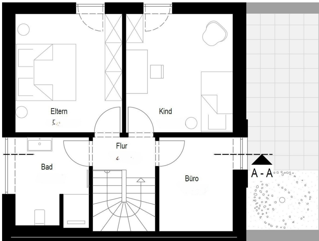
Grundriss Obergeschoss
