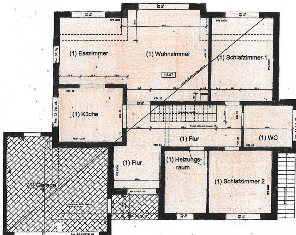
Grundriss Erdgeschoss
