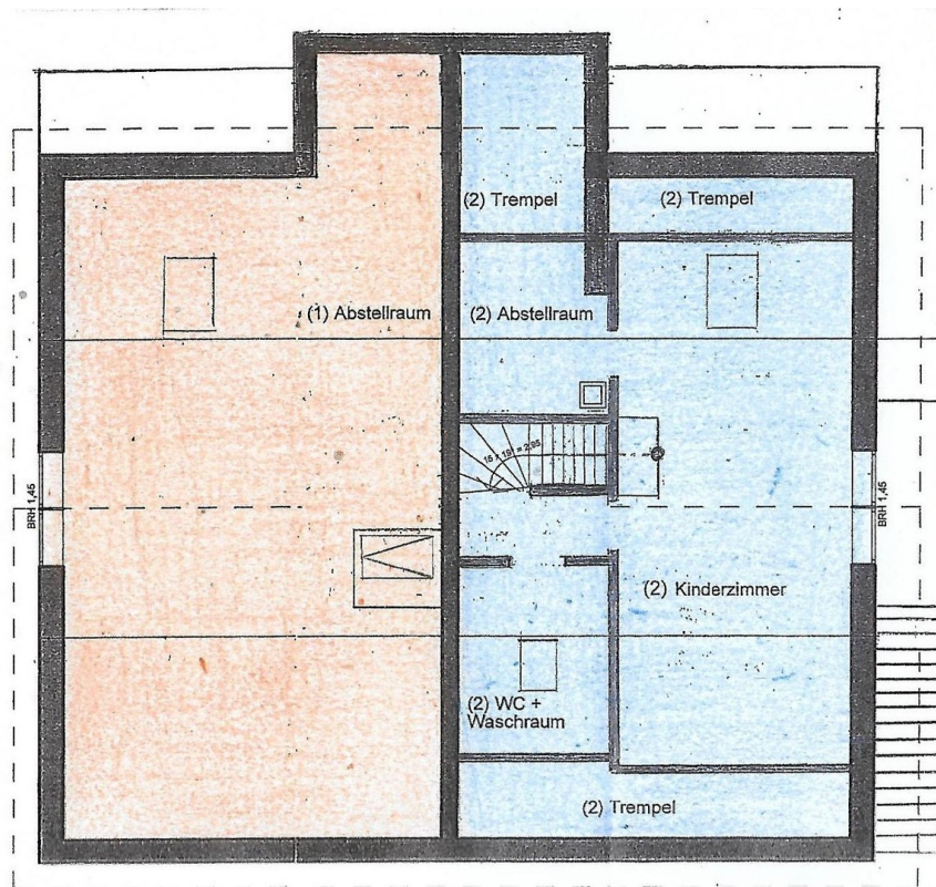
Grundriss Dachgeschoss
