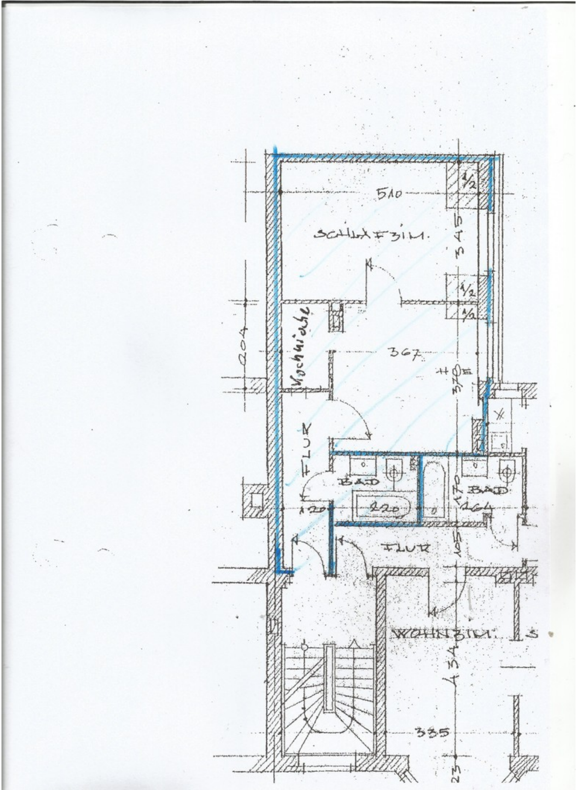
Grundriss 2.OG li
