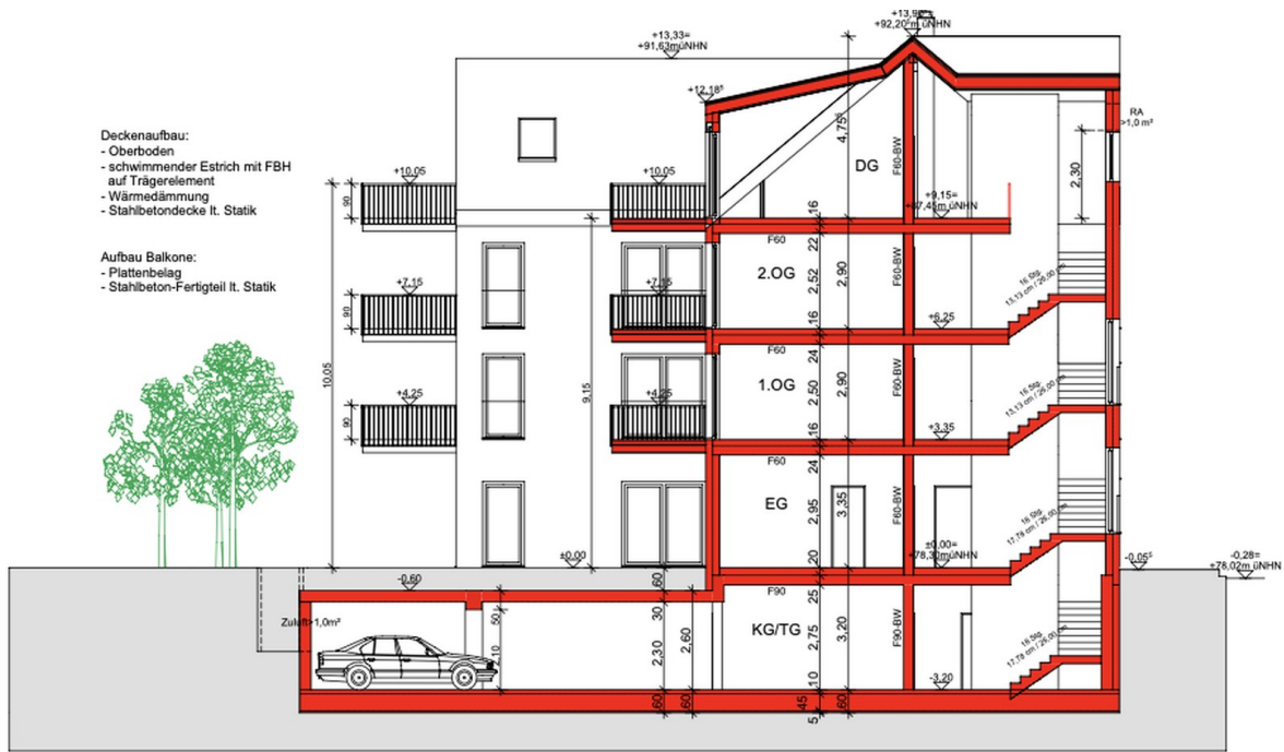
Schnitt B-B
