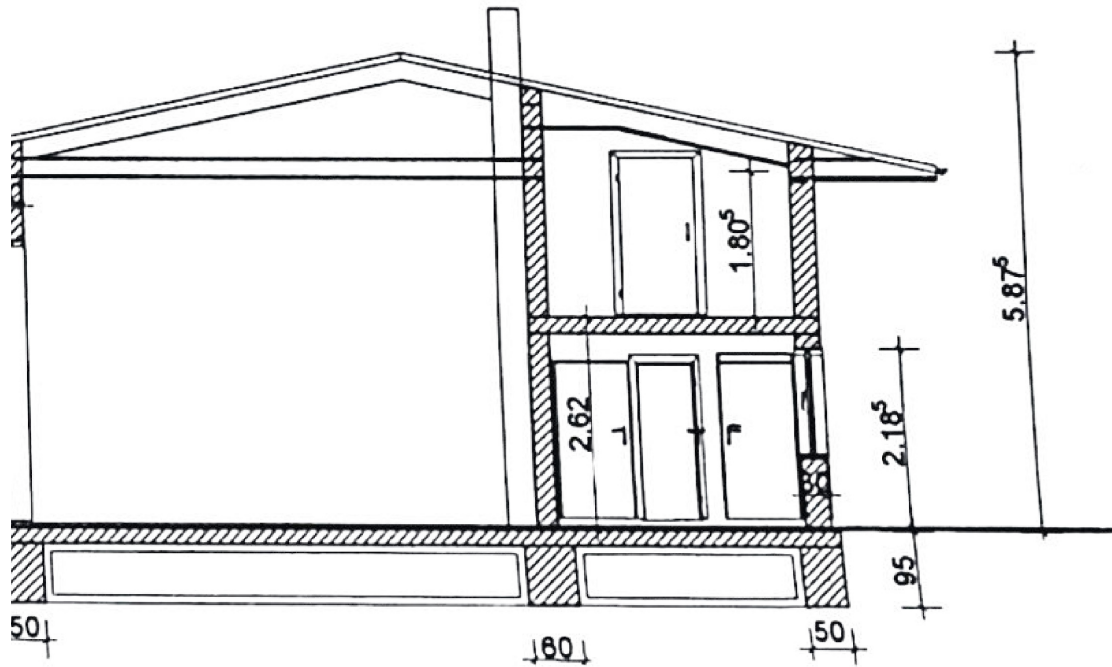
Hallenquerschnitt
