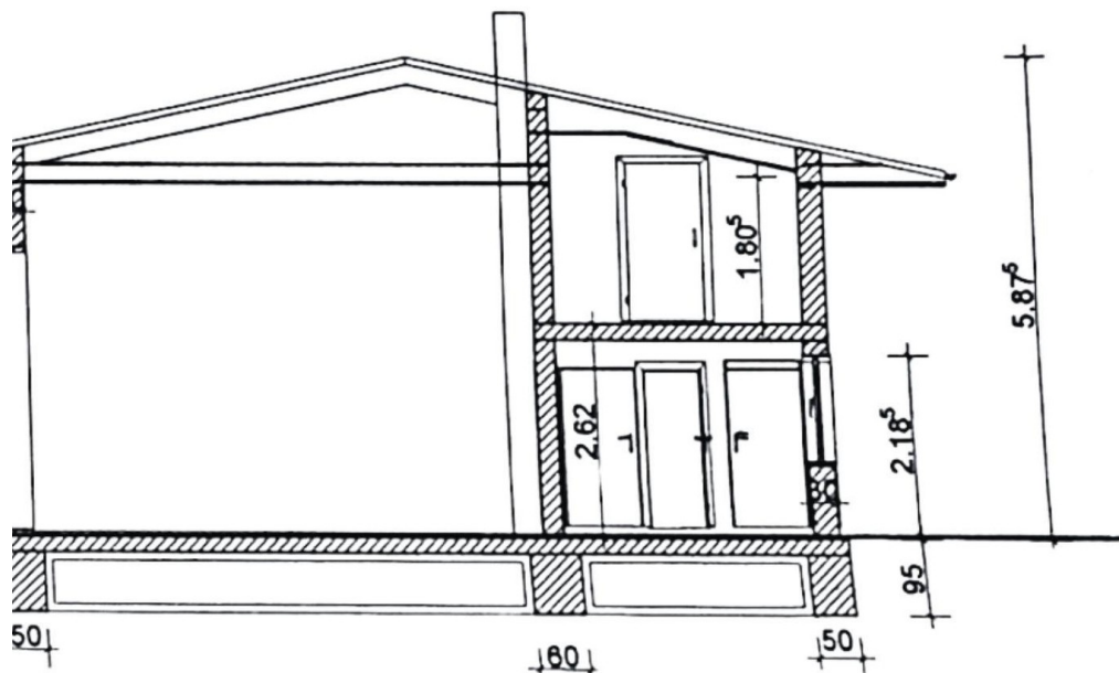
Hallenquerschnitt
