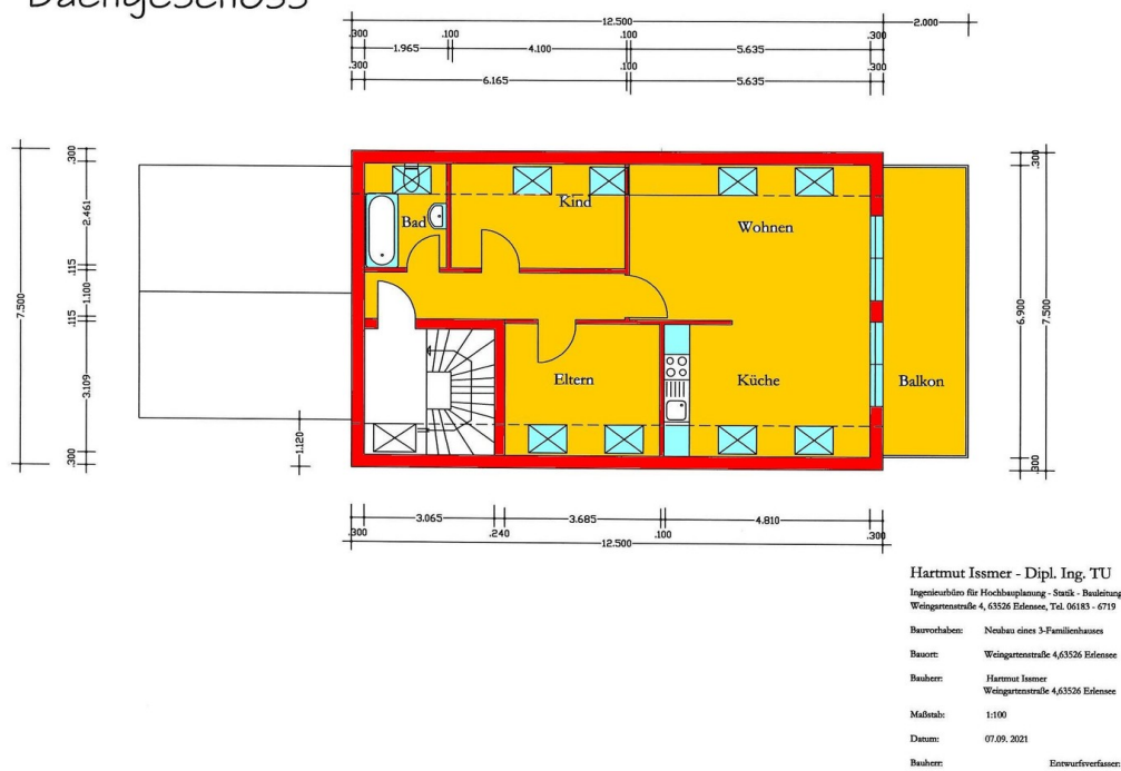
Dachgeschoßgrundriss
