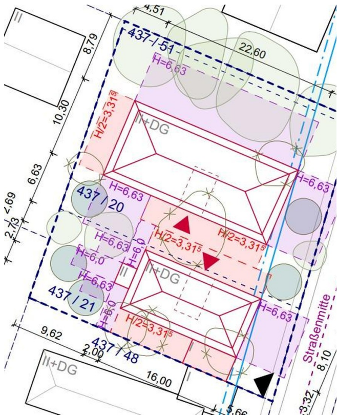
Genehmigte Bebauung
