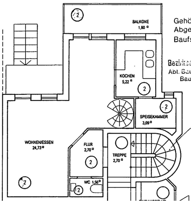
Erdgeschoss Grundriss
