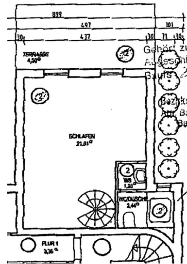
Untergeschoss Grundriss
