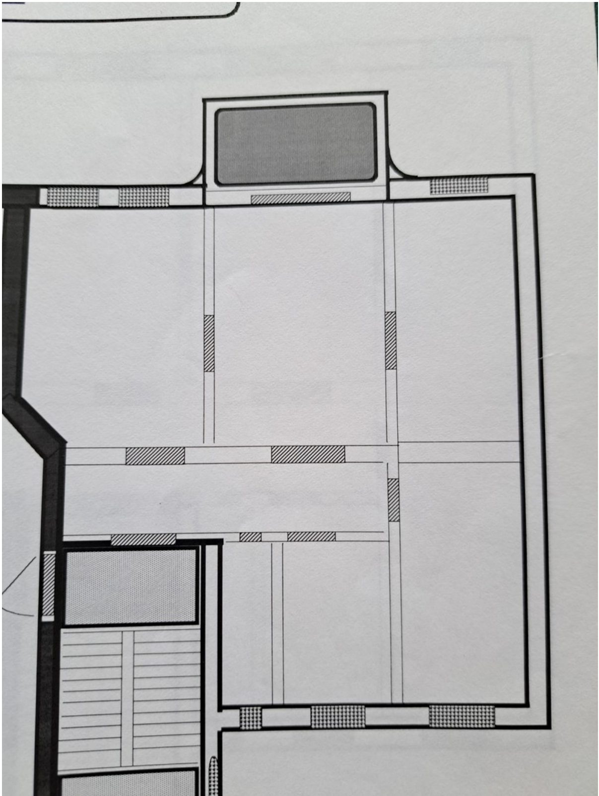
Grundriss Whg 3. OG Ri. Nord
