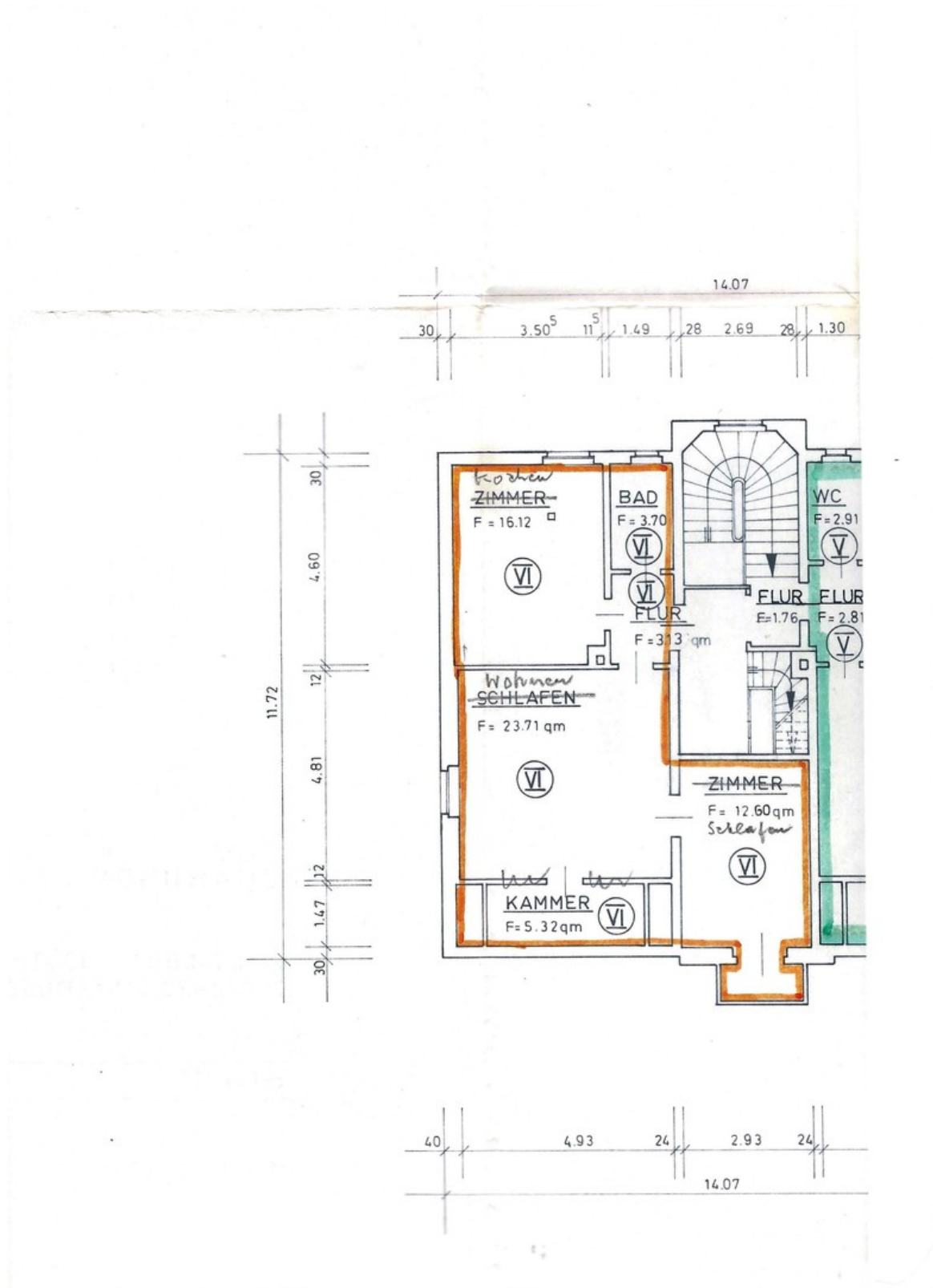
Grundriss DG
