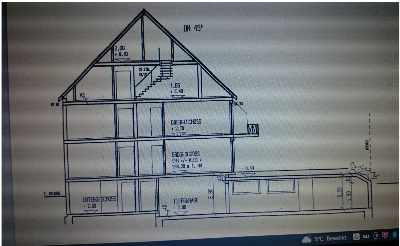
Schnittdarstellung Haus
