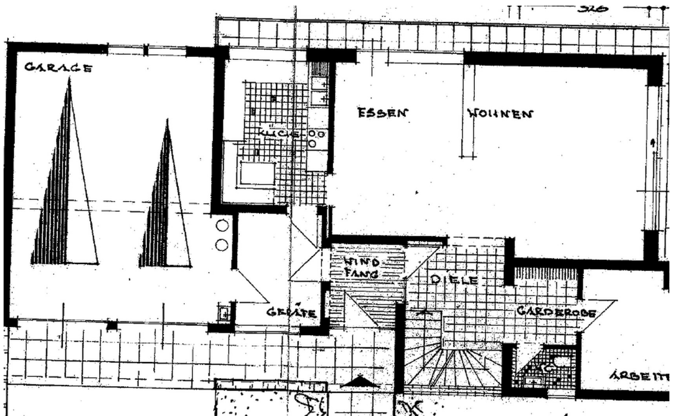
Grundriss EG
