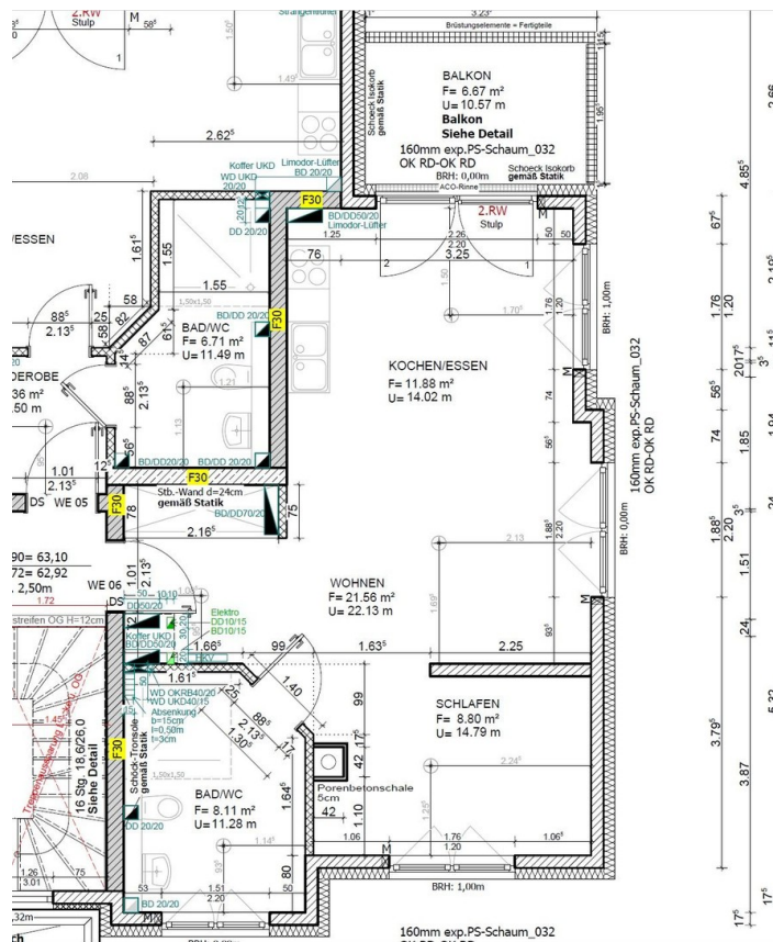
Grundriss
