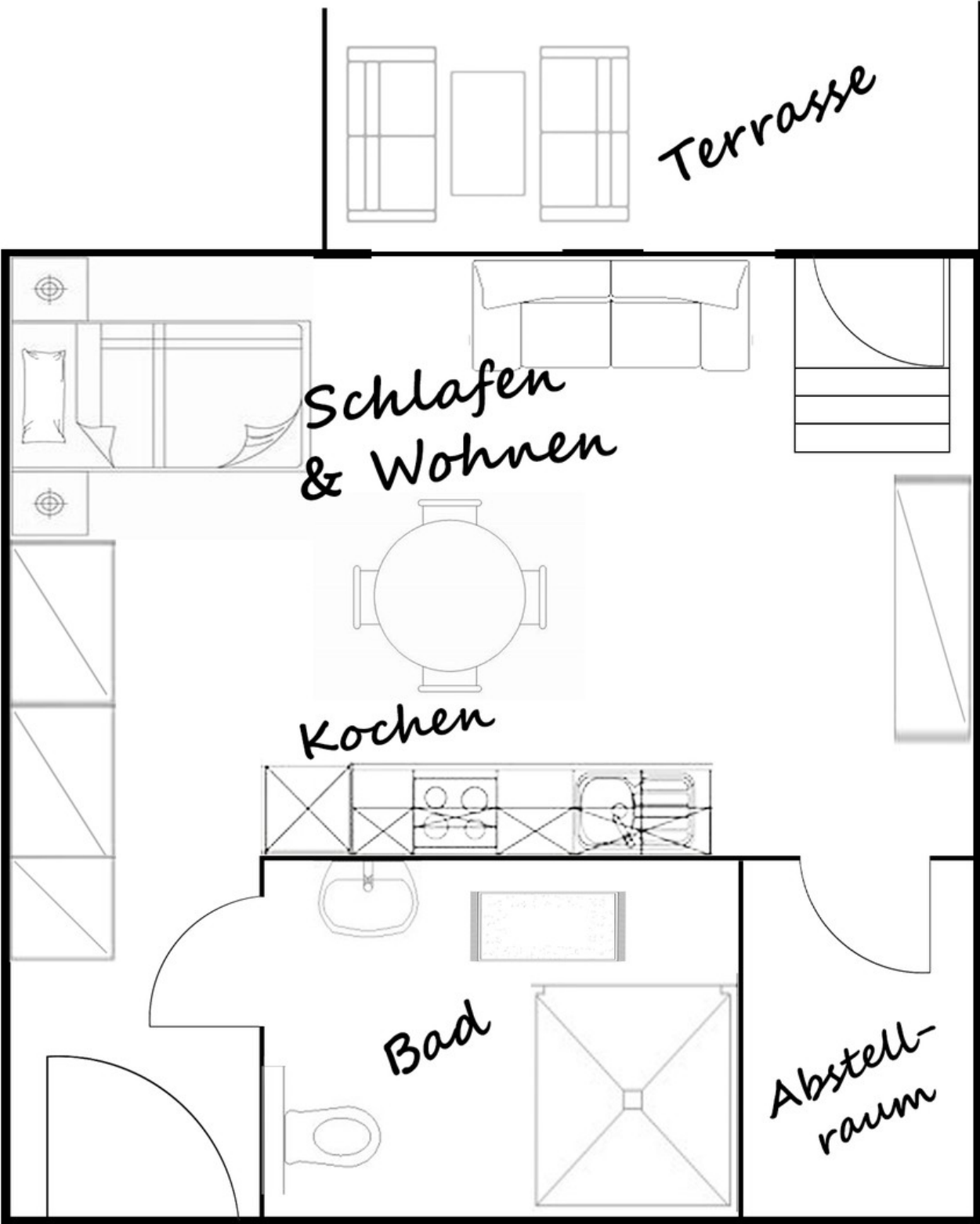
Grundriss
