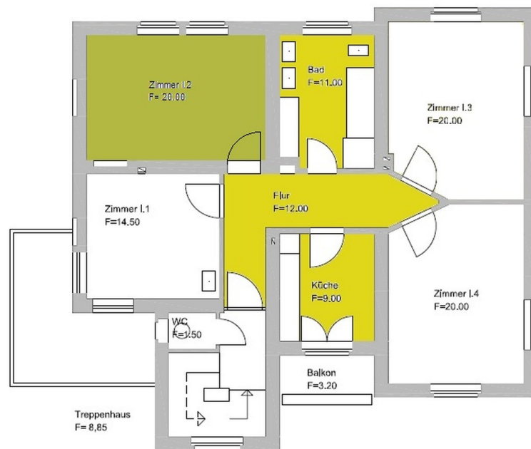
Grundriss 1. Obergeschoss
