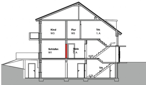
Schnitt A-A 1:100
