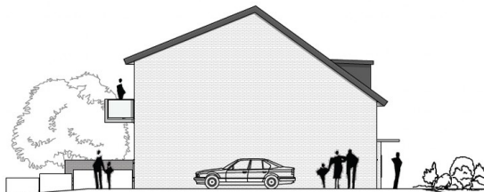
Süd-Ansicht 1:100
