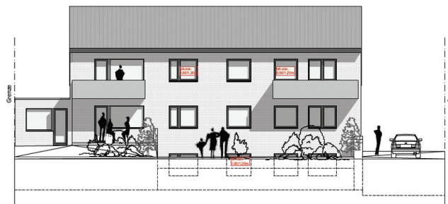
West-Ansicht 1:100
