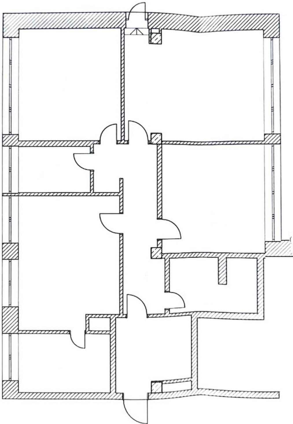
2. OBERGESCHOSS M 1 : 100
