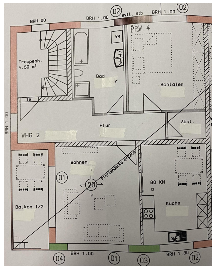
Grundriss OG
