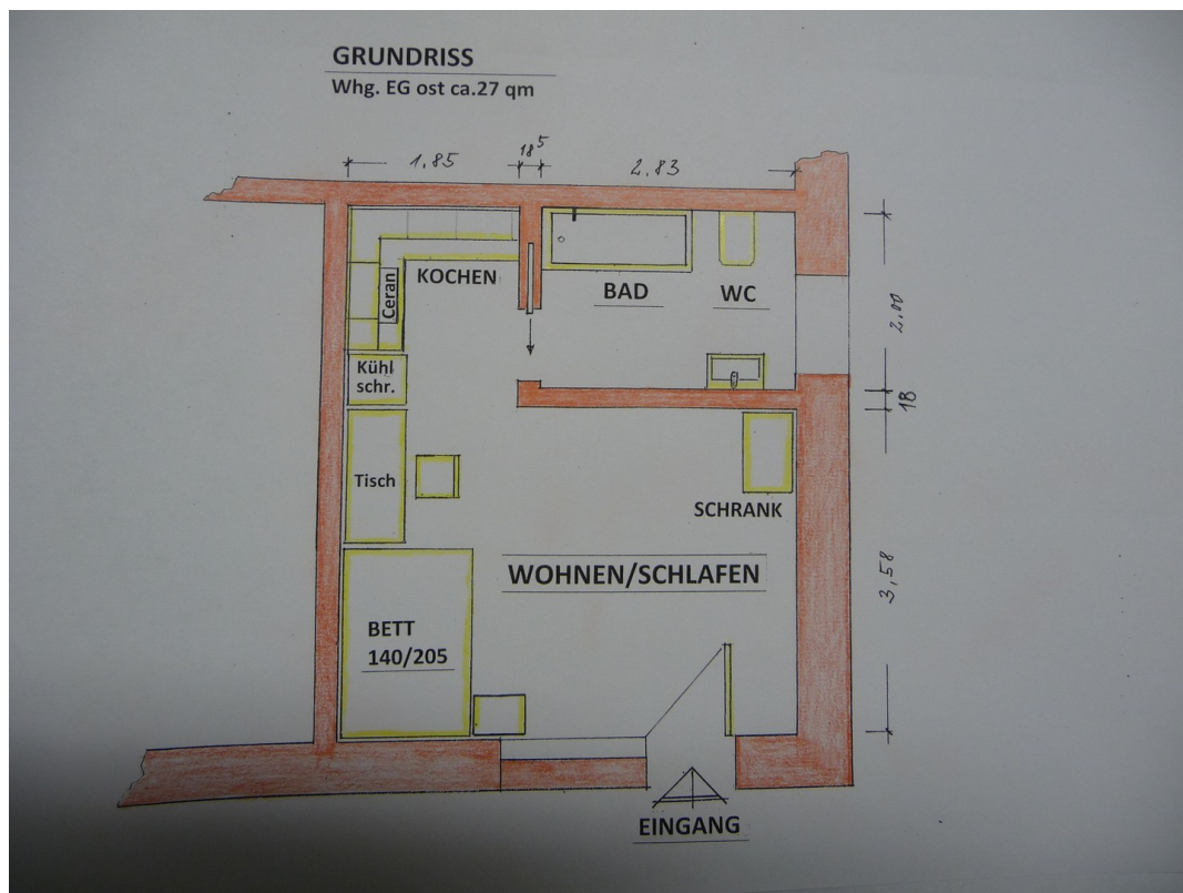
Grundriss EG ost
