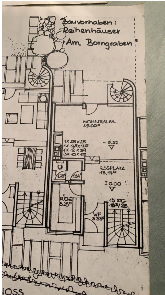
Erdgeschoss
