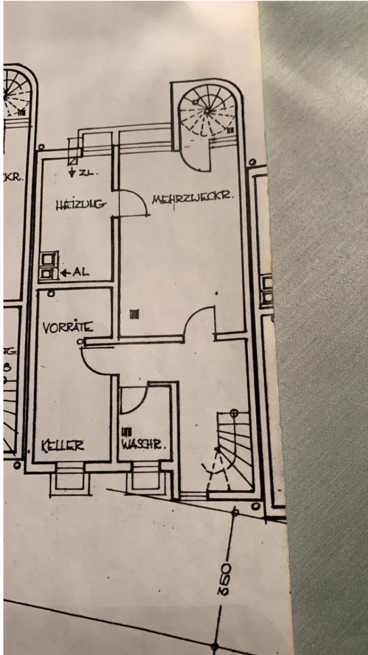
Keller
