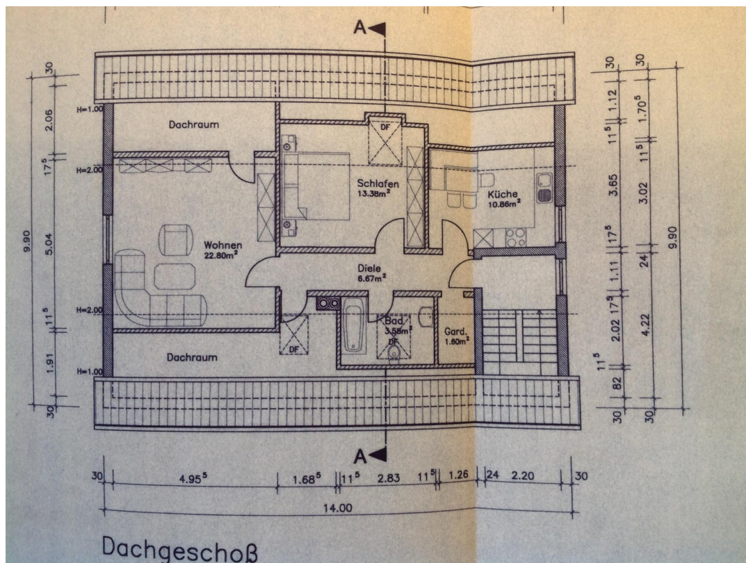
Grundriss DG
