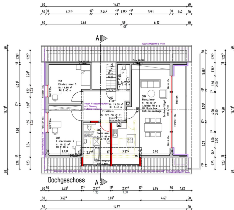
Dachgeschoss
