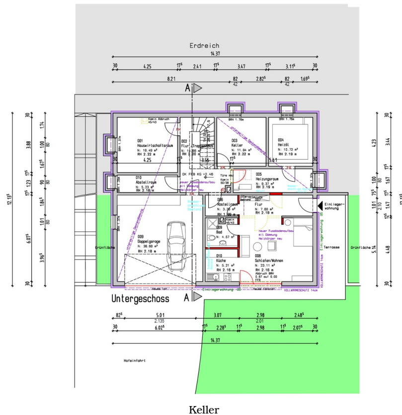
Keller
