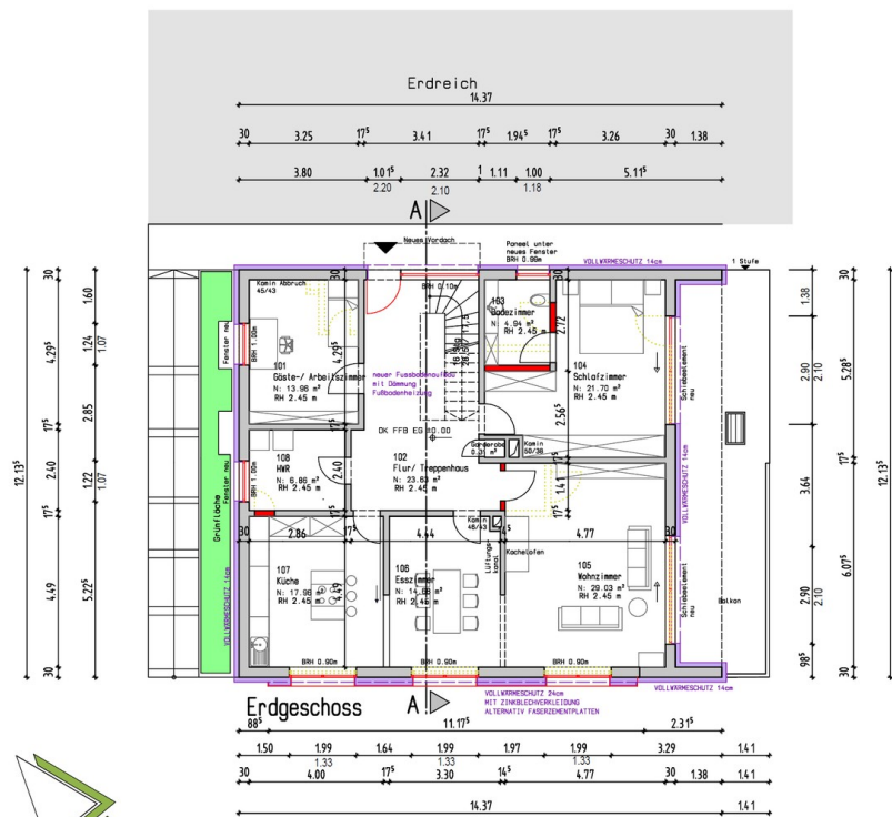
Erdgeschoss
