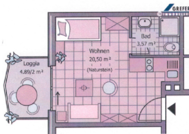
Grundriss
