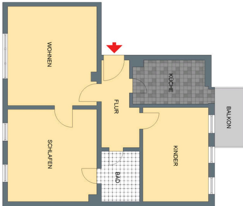
Grundriss
